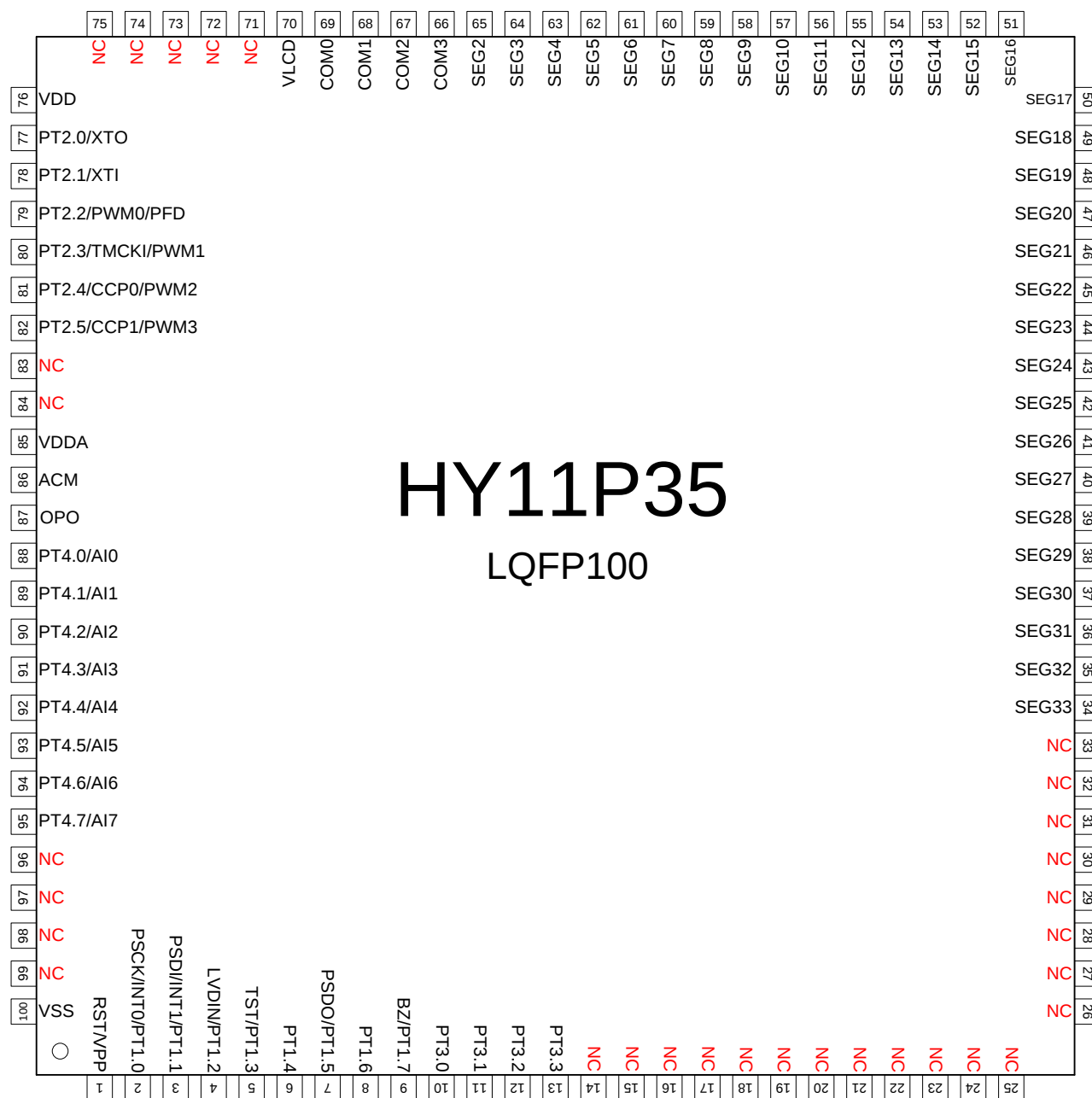
圖 2-1 HY11P35 LQFP100 引腳圖
