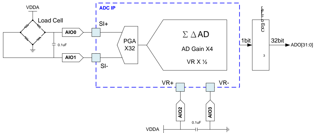
圖 3-4 ADC 電路示意圖
